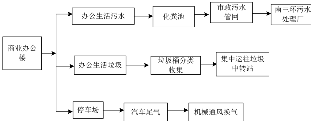
图3 运营期工艺流程及产污环节图
